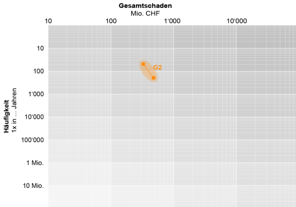
Abbildung 1: Risikodiagramm
