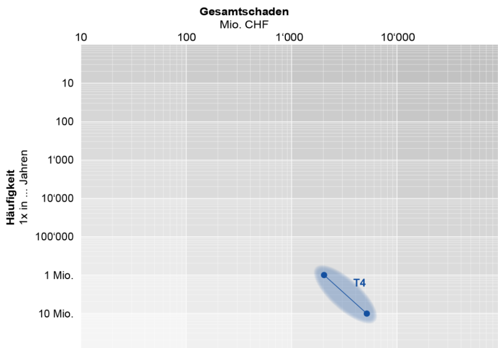
Abbildung 1: Risikomatrix
