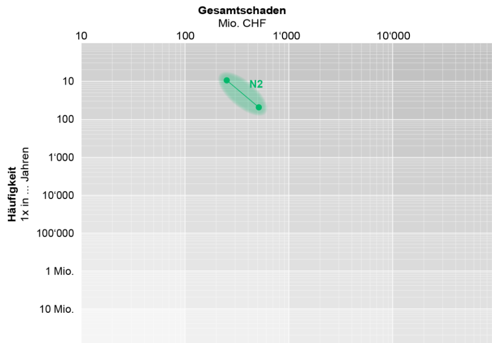
Abbildung 1: Risikomatrix
