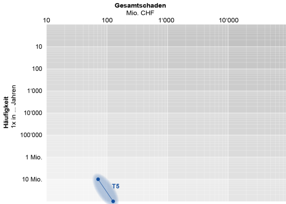
Abbildung 1: Risikomatrix
