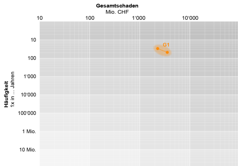
Abbildung 1: Risikodiagramm
