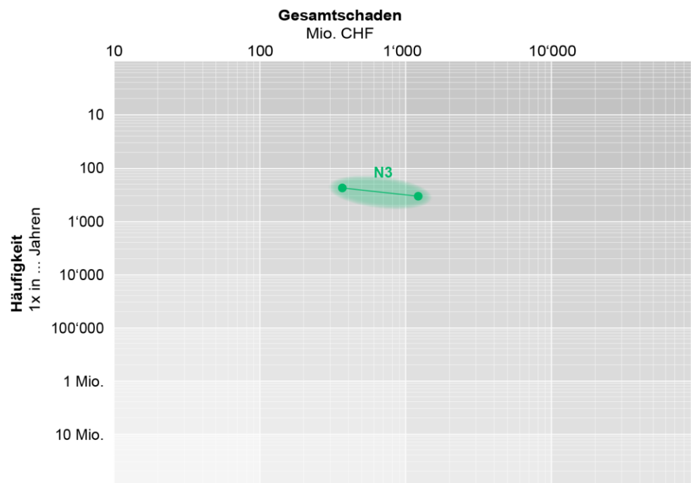
Abbildung 1: Risikomatrix
