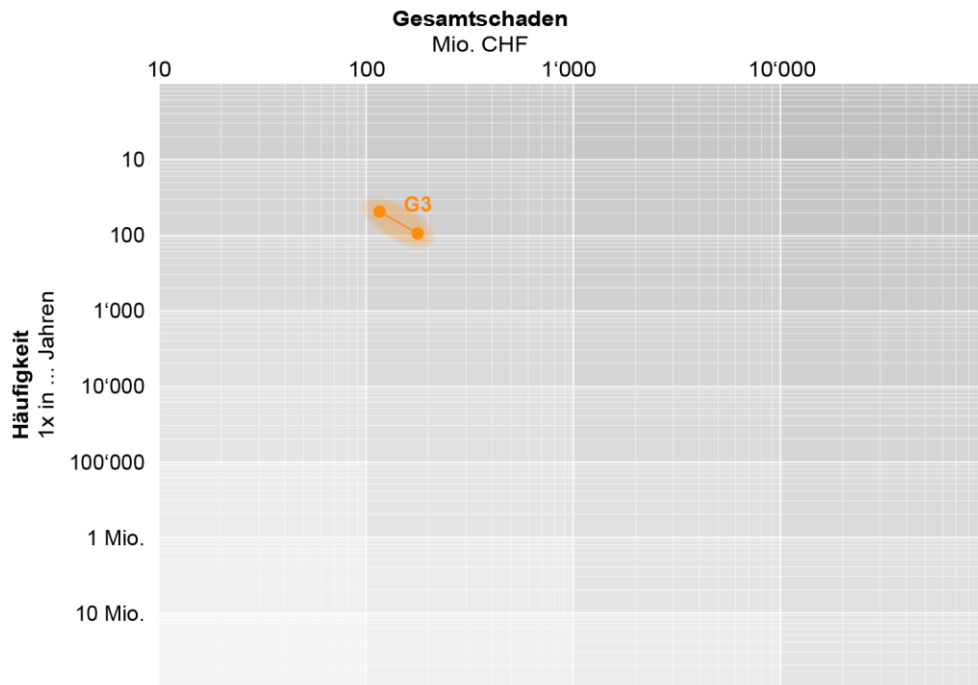
Abbildung 1: Risikomatrix
